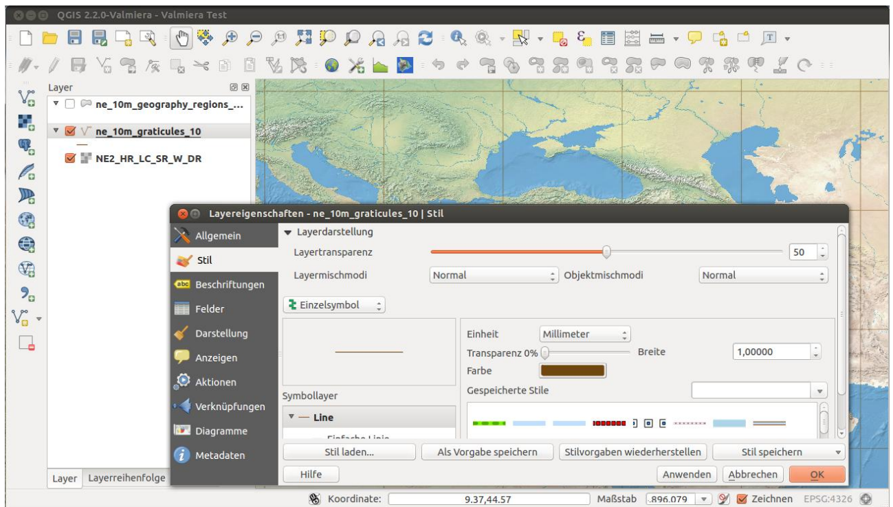
Рис. 1.3 – інтерфейс QGIS
